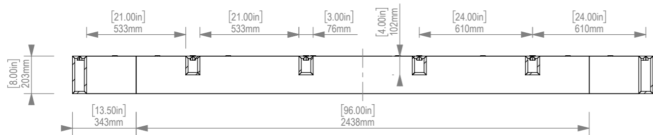
SECTION A-A
